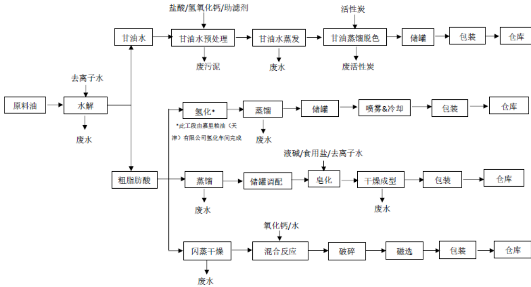
图 1 工艺流程图
